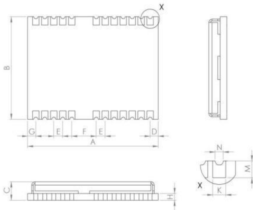
图3-1 SKG4303D模块封装尺寸示意图
