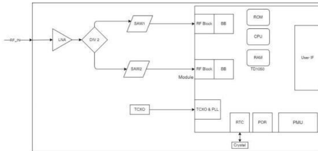
1-2 模块功能框图
