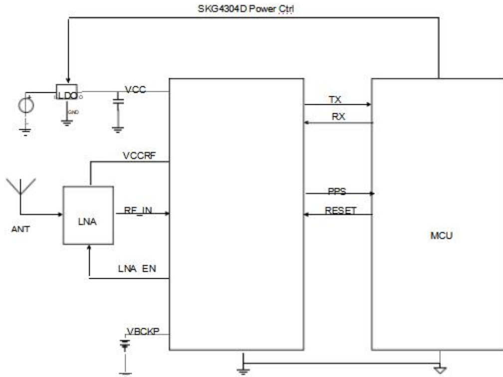
图 1-3 SKG4303D 模块典型应用图
