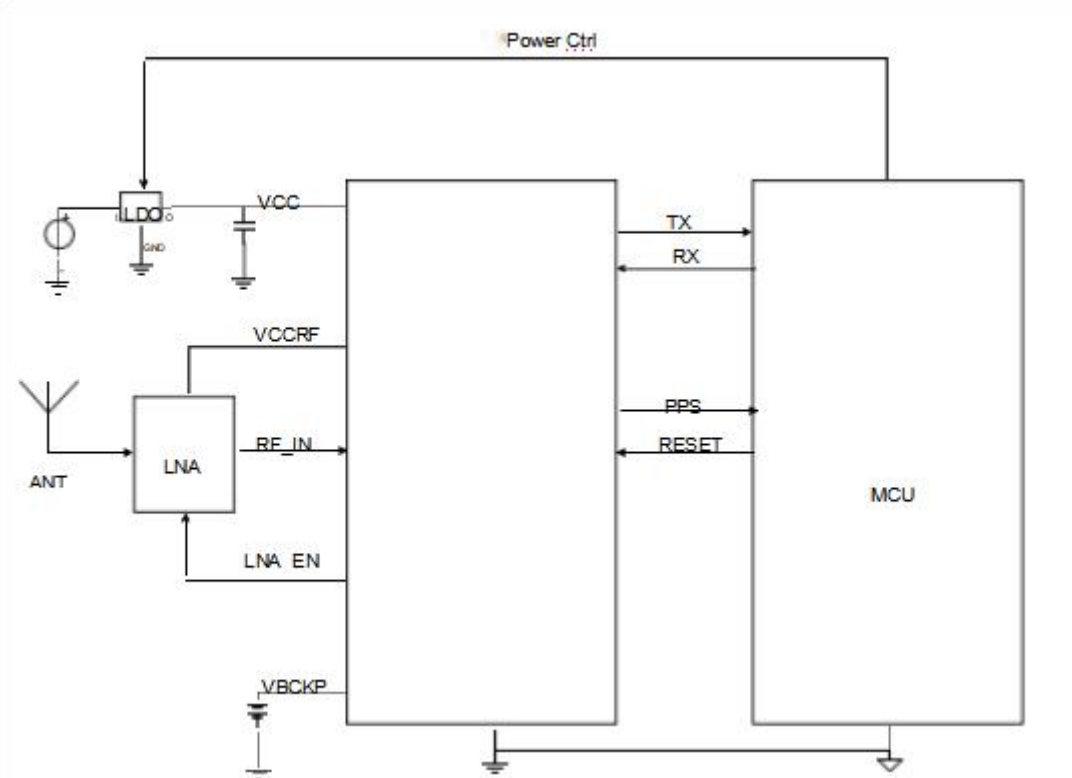
图 1-3 SKG12D-09 模块典型应用图
