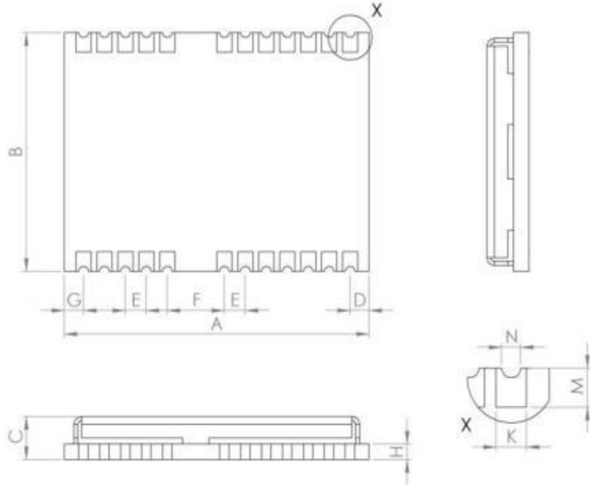
图 3-1 SKG12D-09模块封装尺寸示意图
