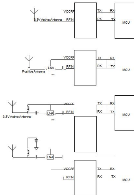
图 2-1 天线供电的几个不同应用示意图
