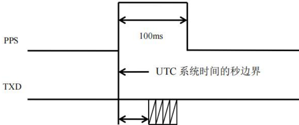
图 2-3 1PPS 秒脉冲示意图
