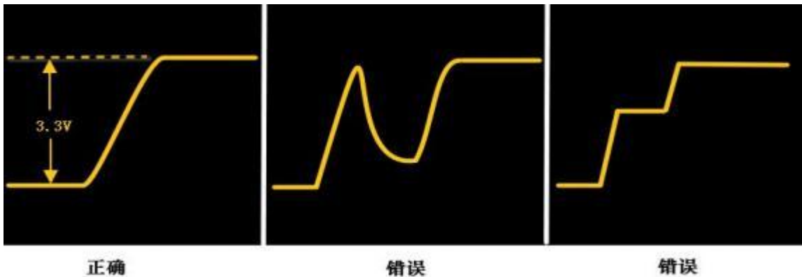
图5-1 主电上电示意图
