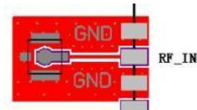
图 5-2 第 11 脚 RF_IN 连接线设计示意图
