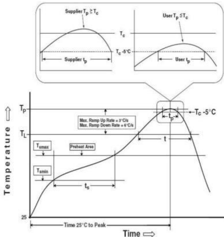
图 4 SKG8203B模块贴装回流焊曲线示意图
