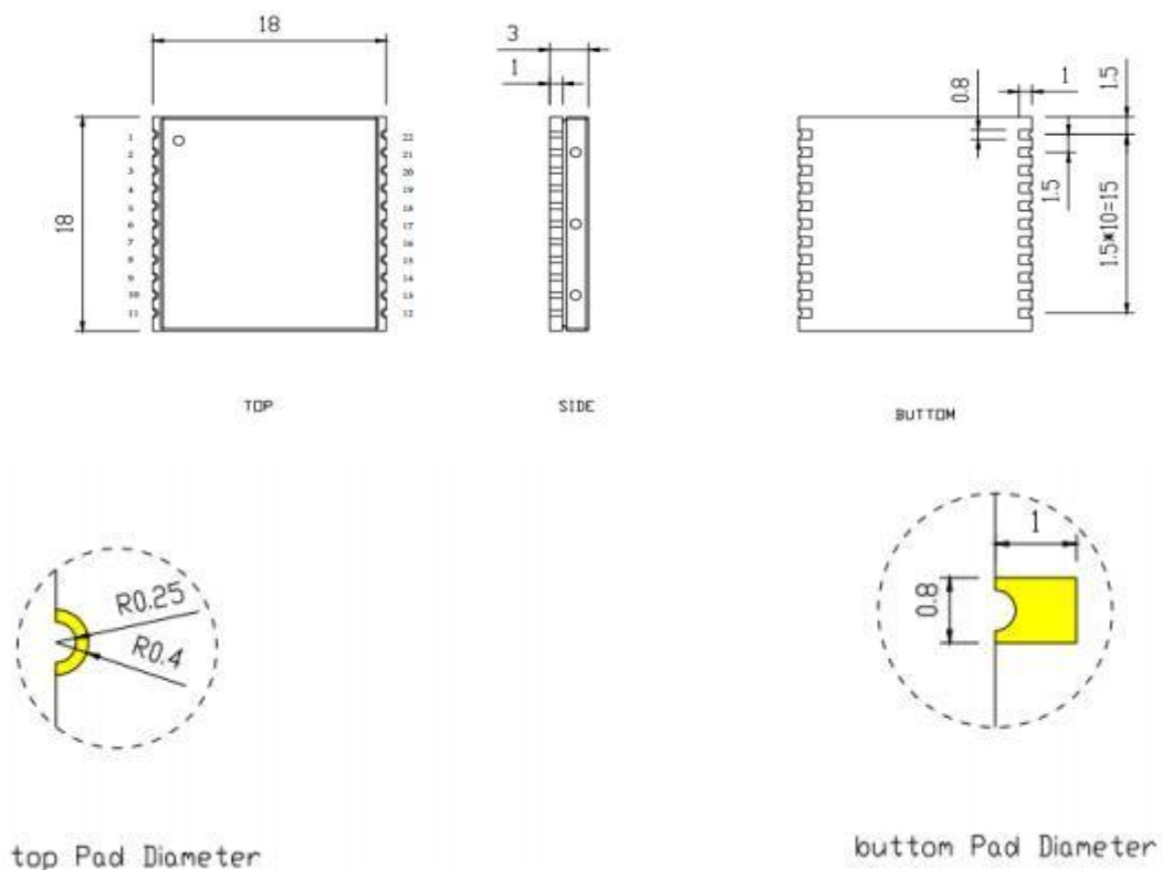
图 2 SKG8203B模块封装尺寸示意图
