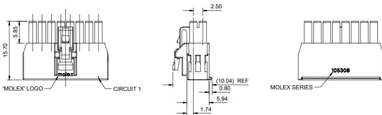
图 4: MOLEX 连接头 105308-1206 尺寸
