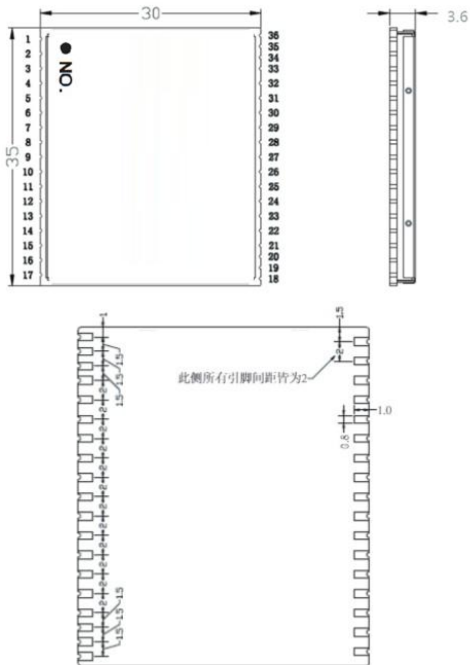
图 2 SKG30AX-09H 模块封装尺寸示意图
