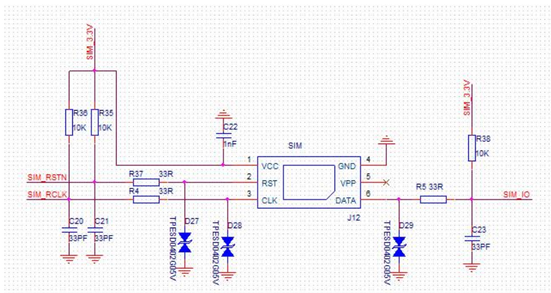
图 3 SKG30AX-09H 模块原理设计参考图
