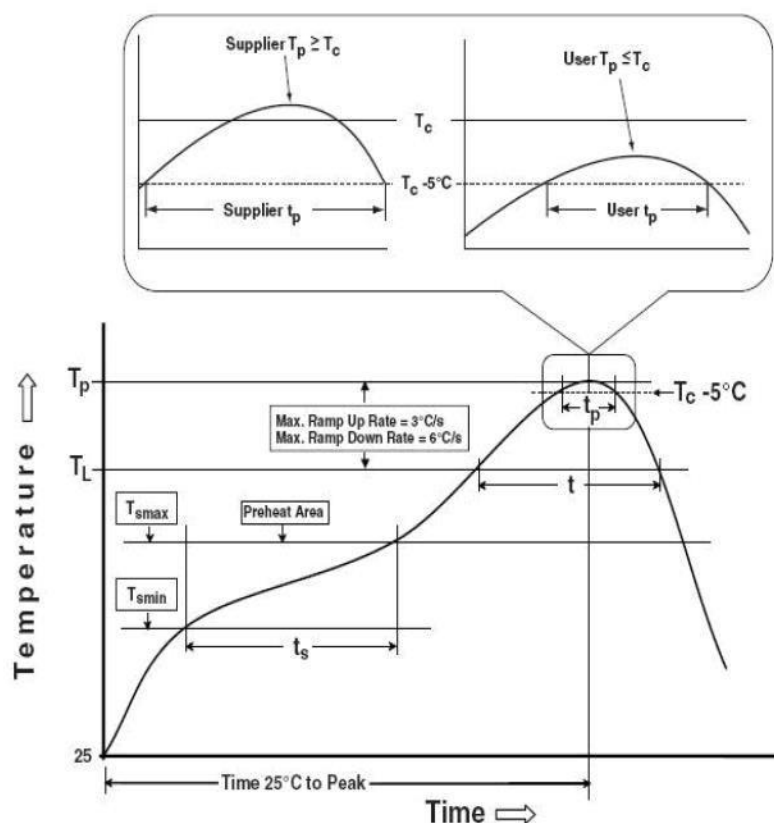
图 4 SKG30AX-09H 模块贴装回流焊曲线示意图
