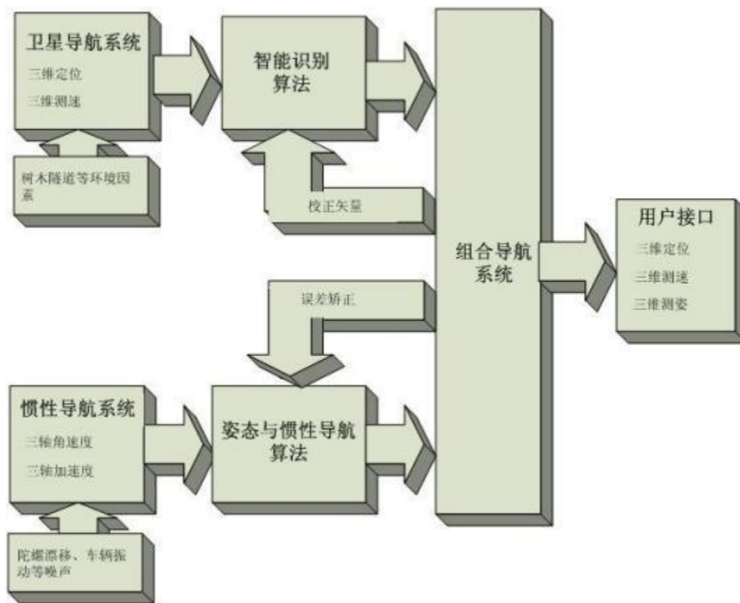
图 3: SKM4507MR-50FXT 设计原理框图/Design diagram
