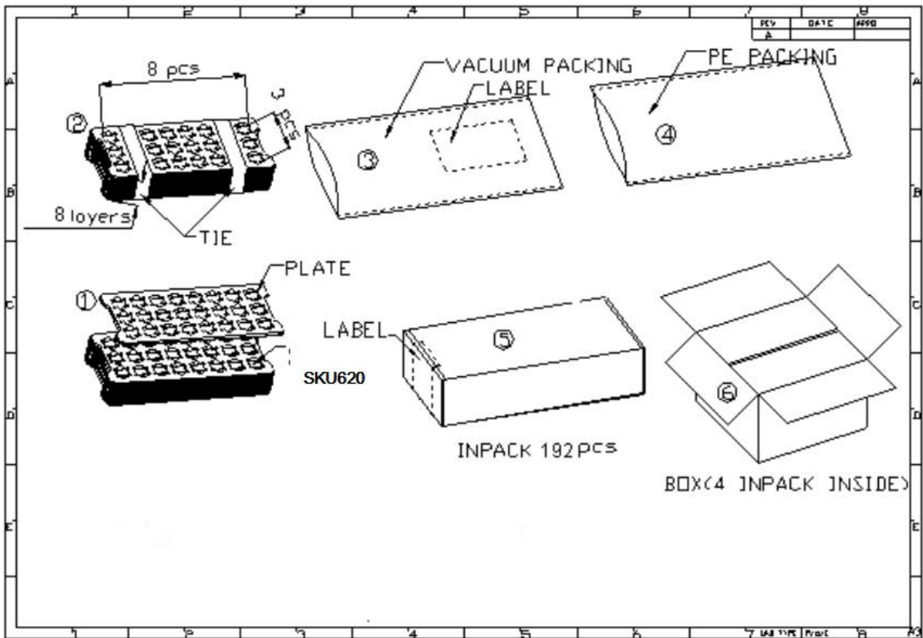
Figure10-1: SKU623 Packaging
