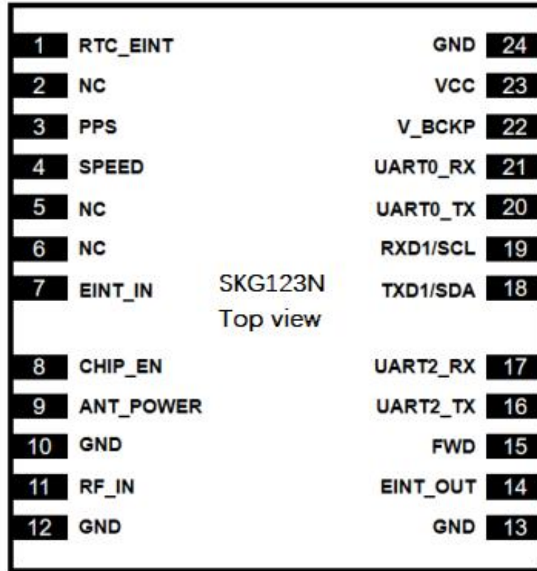
图 2: SKG123NR 管脚定义/pin definitions
