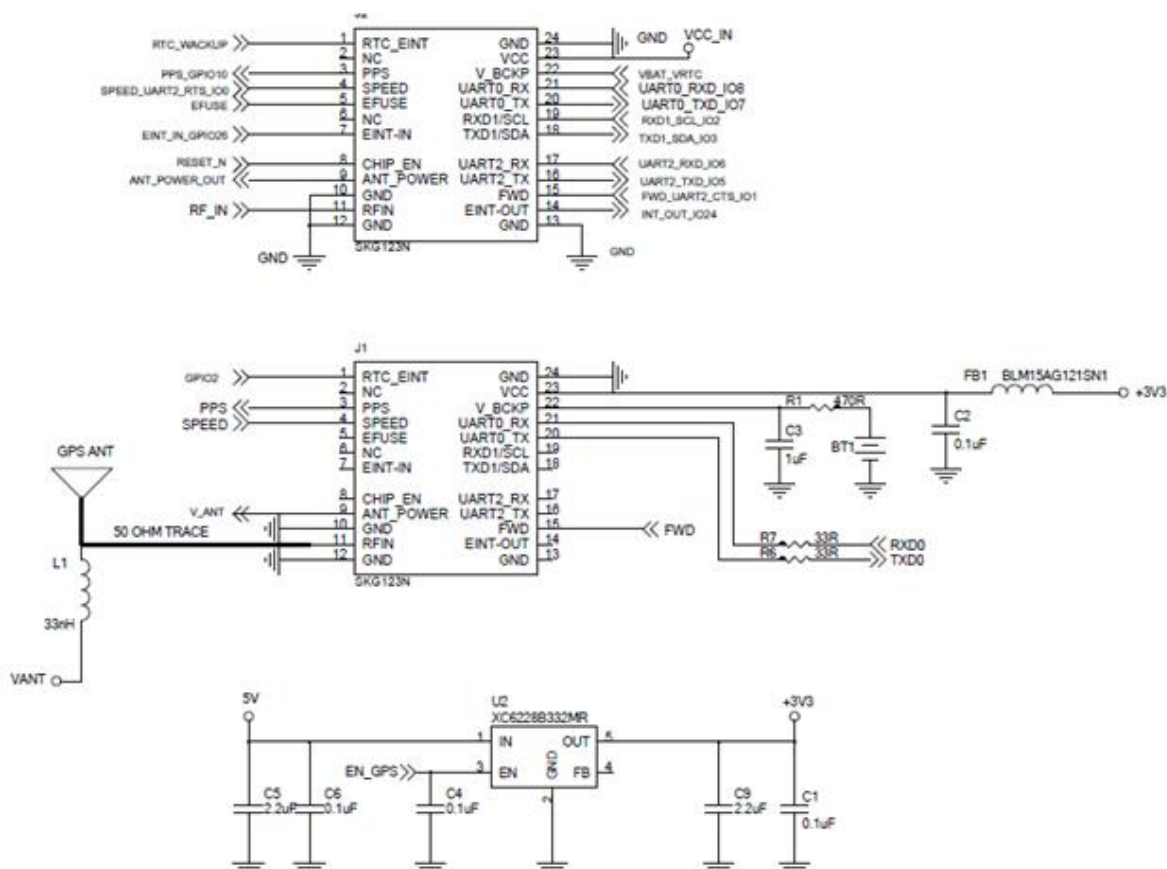
图 4: SKG123NR 参考电路//Reference circuit
