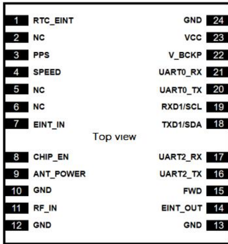
图 2: SKG123ND 管脚定义/pin definitions
