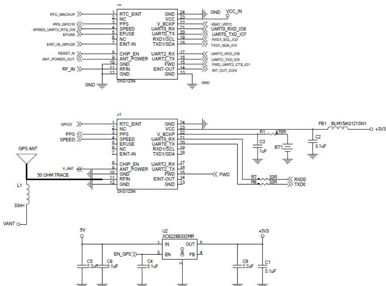
图 4: SKG123ND 参考电路//Reference circuit
