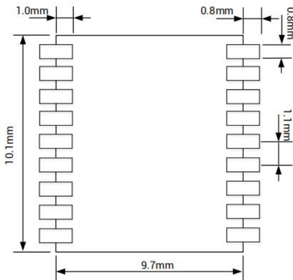
图 6：封装参考
