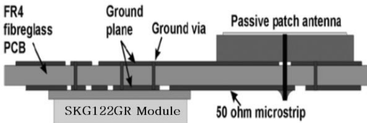
图 11.1-1 SKG122GR 参考设计/ Figure 11.1-1 SKG122GR reference design
